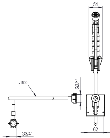
Front aanzicht
